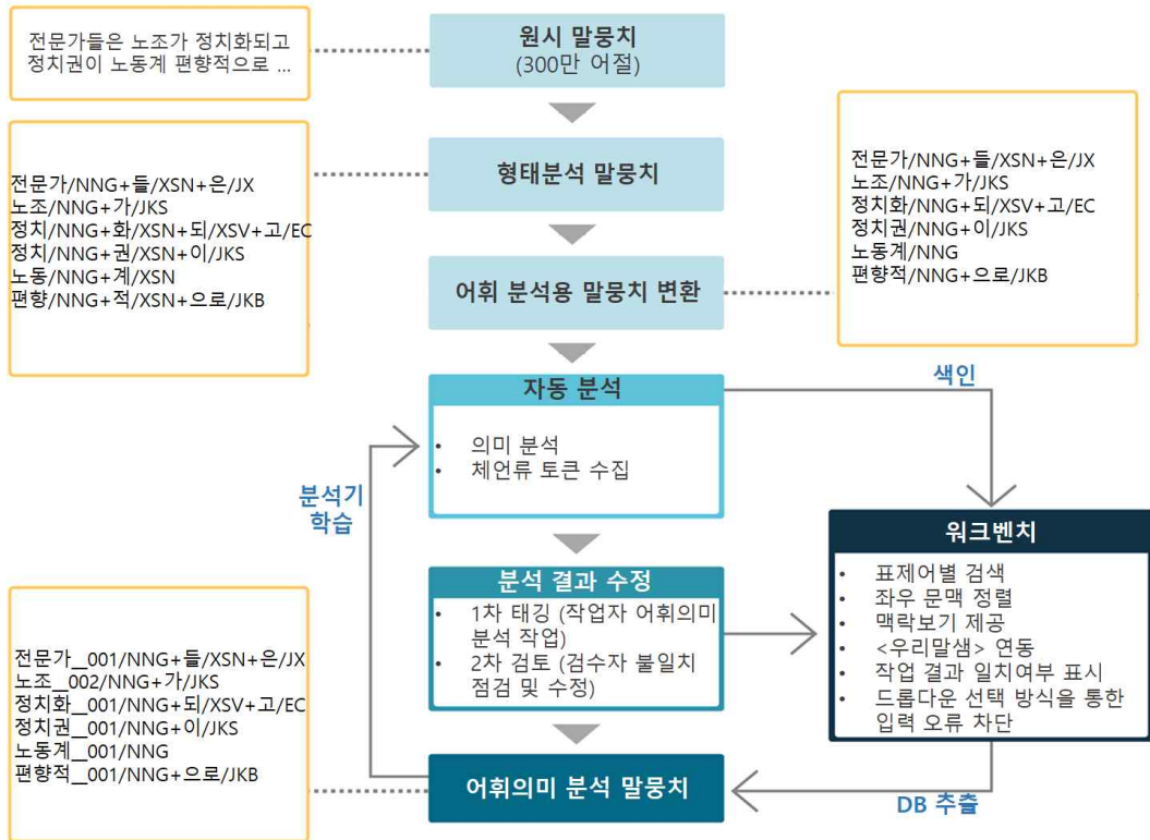
<그림 1> 어휘의미 말뭉치 구축 과정
