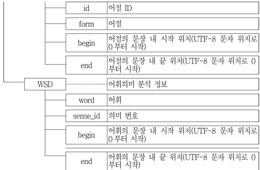
<표 12> JSON 형식의 기본 구조
